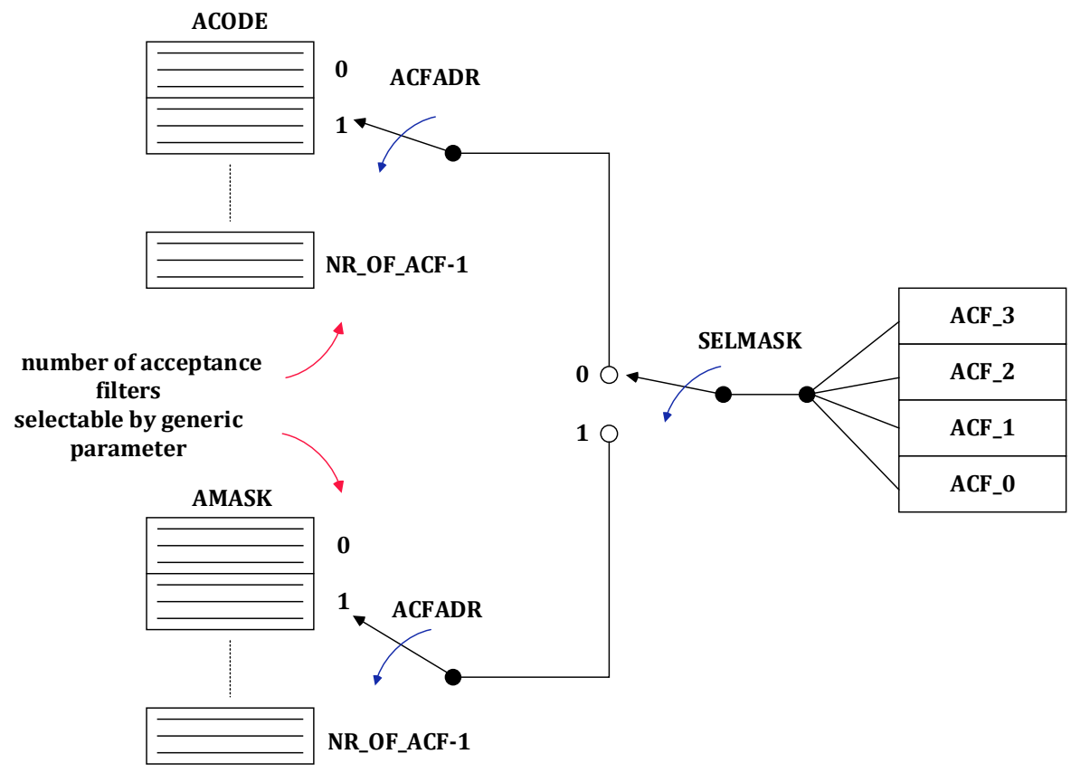
图 21-7 接收过滤器
