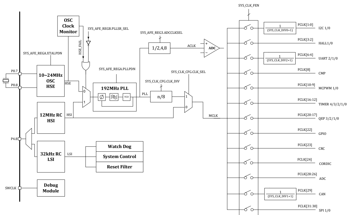
图 6-1 时钟架构
