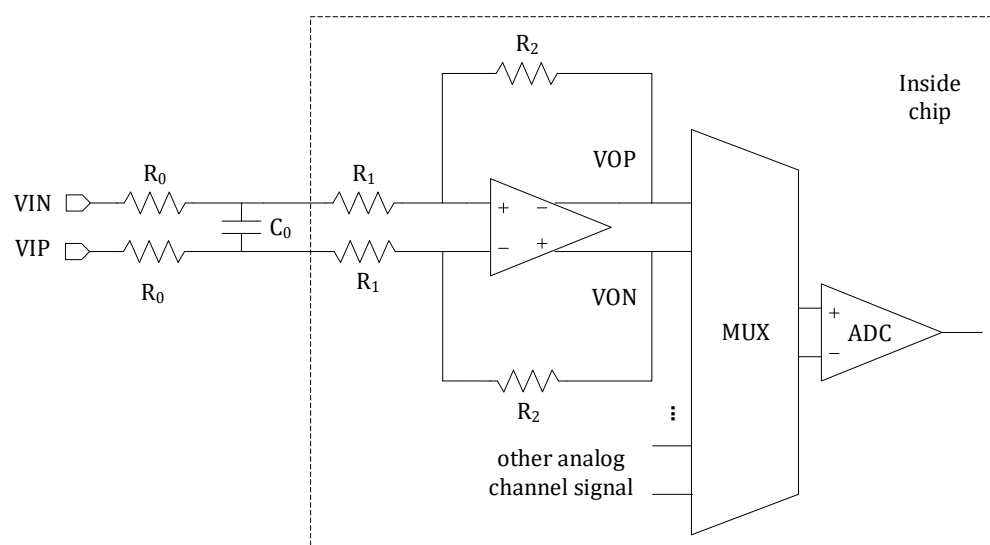
图 5-2 放大器框图
