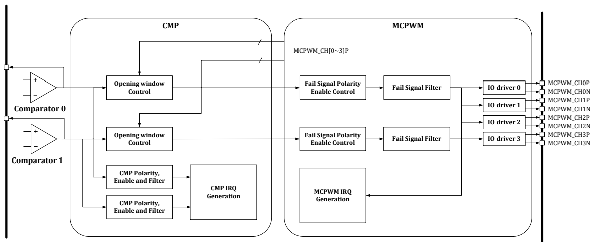
图 20-3 CMP 与 MCPWM 的联动
