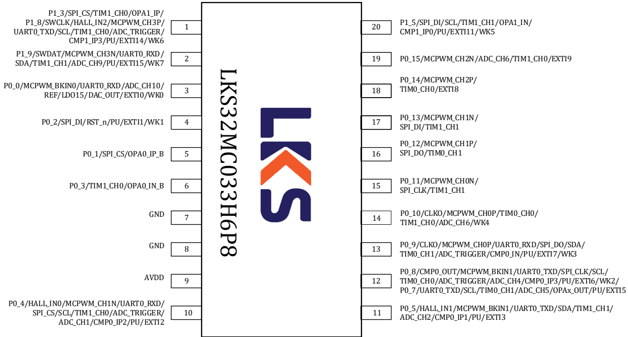
图 3-2 LKS32MC033H6P8 管脚分布图
