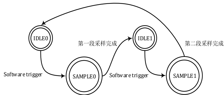
图 12-4 ADC 两段采样状态转移图
